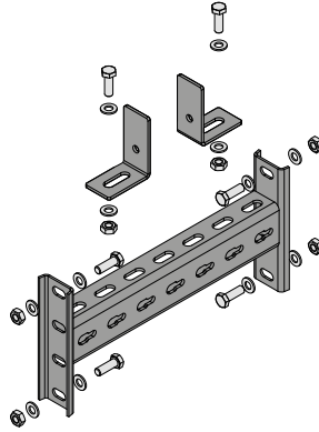
CCR/CR-UT Askı Takımı ("T" cıvatasız)
