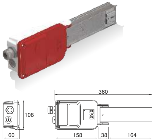
Sondan Besleme
