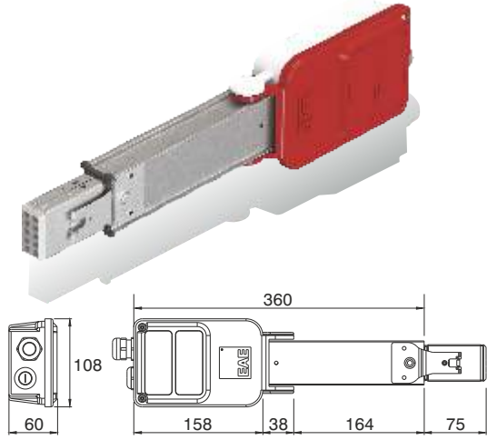
Baştan Besleme
