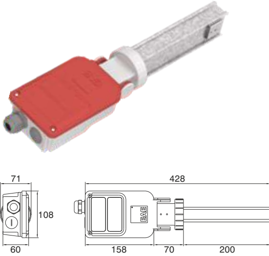
Baştan Besleme
