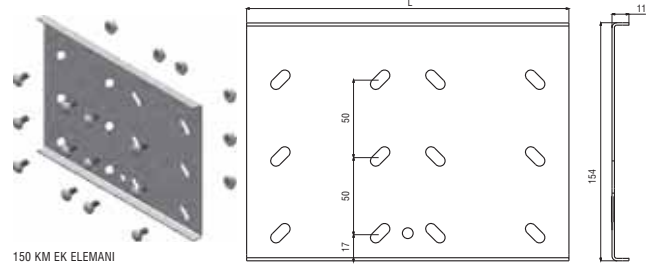
150 KM EK ELEMANI
