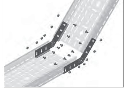
4 Adet Seviye Değiştirme Elemanı, 4 Adet M6x12 Cıvata, 4 Adet M6 Somun içerir.
