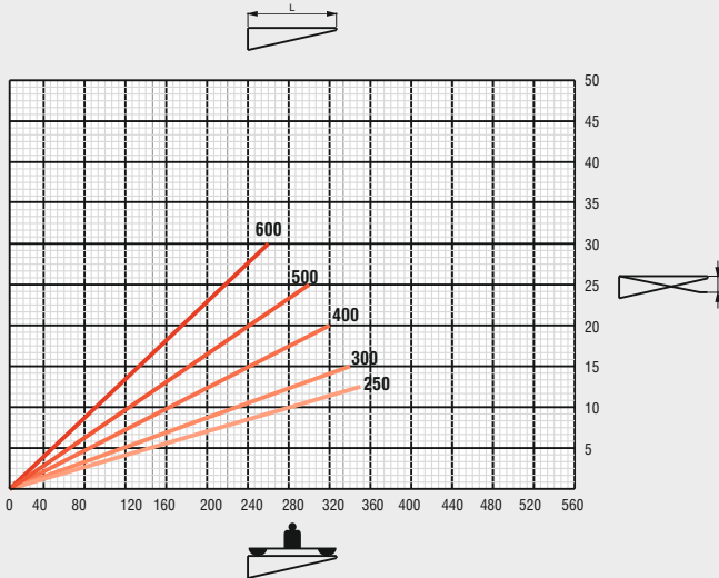
STK MAX YÜK ve SEHİM DEĞERLERİ
