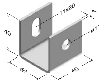
"U" Tavan Tespit Elemanı
