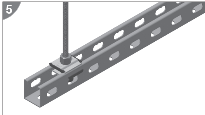
5. Konumu belirlenen hızlı Somunu sıkıştırarak sabitleyiniz..
