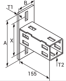
Açılı Tutucu Dikey Bağlantı
