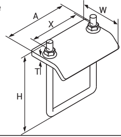
Kiriş Sabitleme U Bolt
