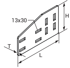
Köşe Tutucu Plaka - Yatay
